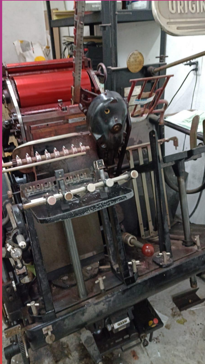
HEIDELBERG FOLIADORA TAMAÑO OFICIO
